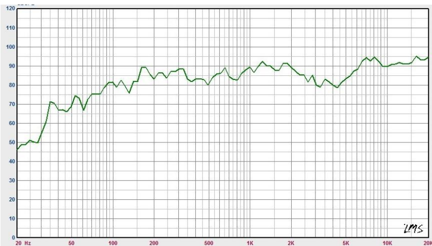
Frequenzbereichkurve: (dB SPL im Vergleich zur Frequenz)
