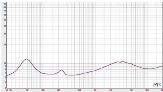
Grafico dell'impedenza:
