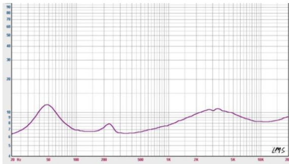
Diagramme d'impédance :
