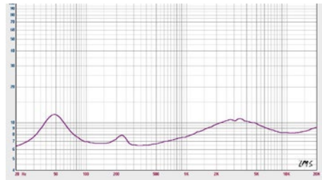
Impedanz-Kurve:
