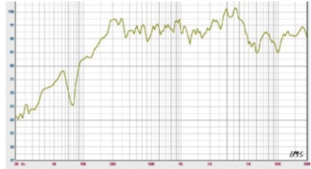
Frequenzgang-Kurve:
